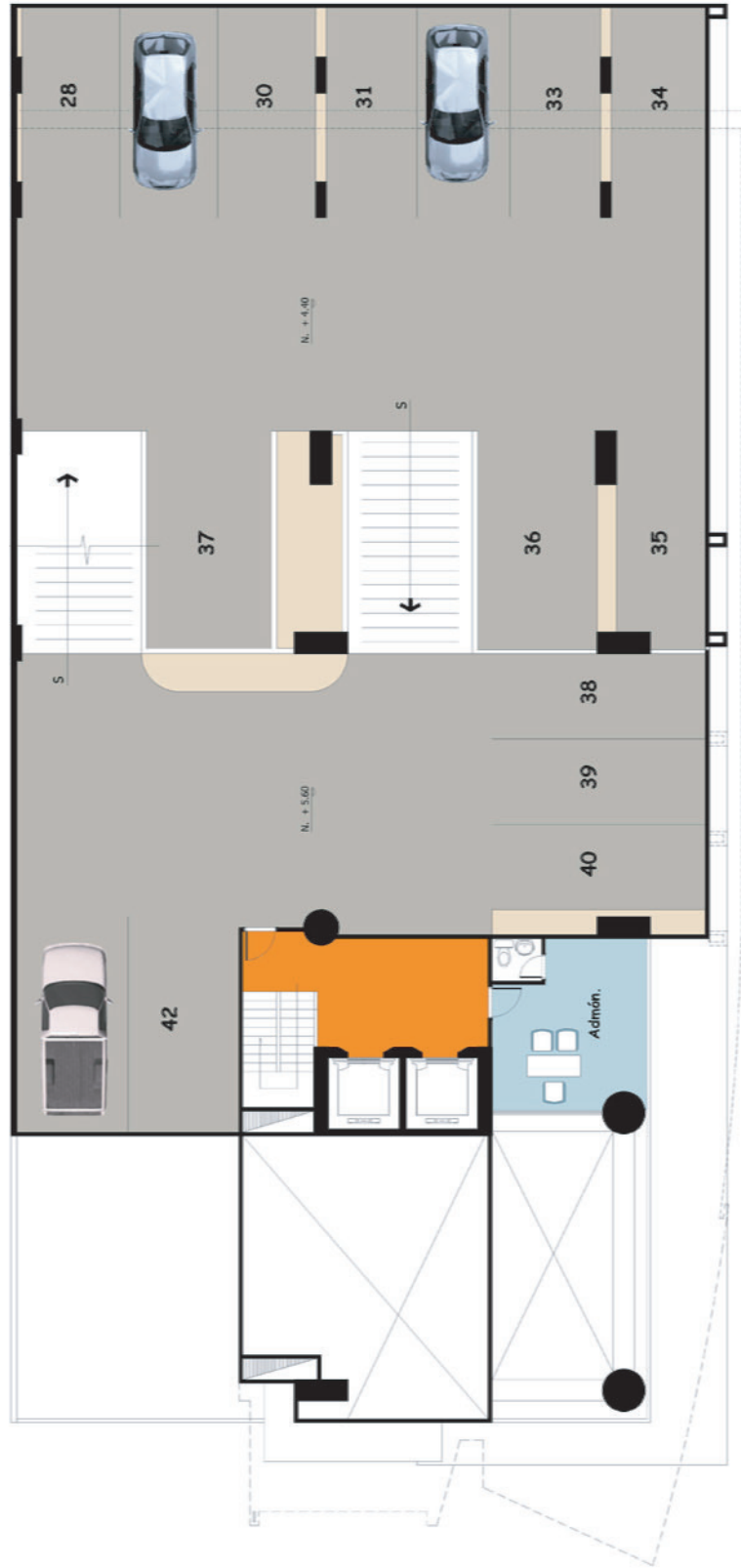
PLANTA NIVEL + 4.40 + 5.60
