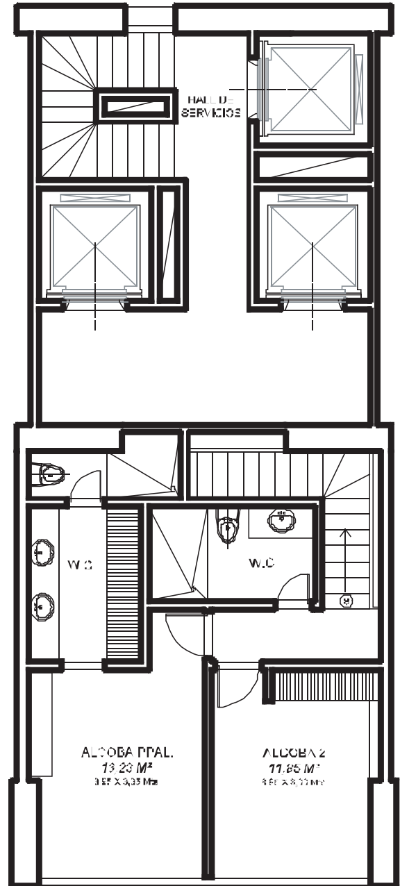
PLANTA BAJA
