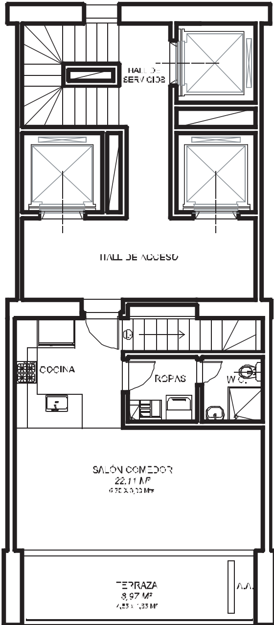
PLANTA ALTA
